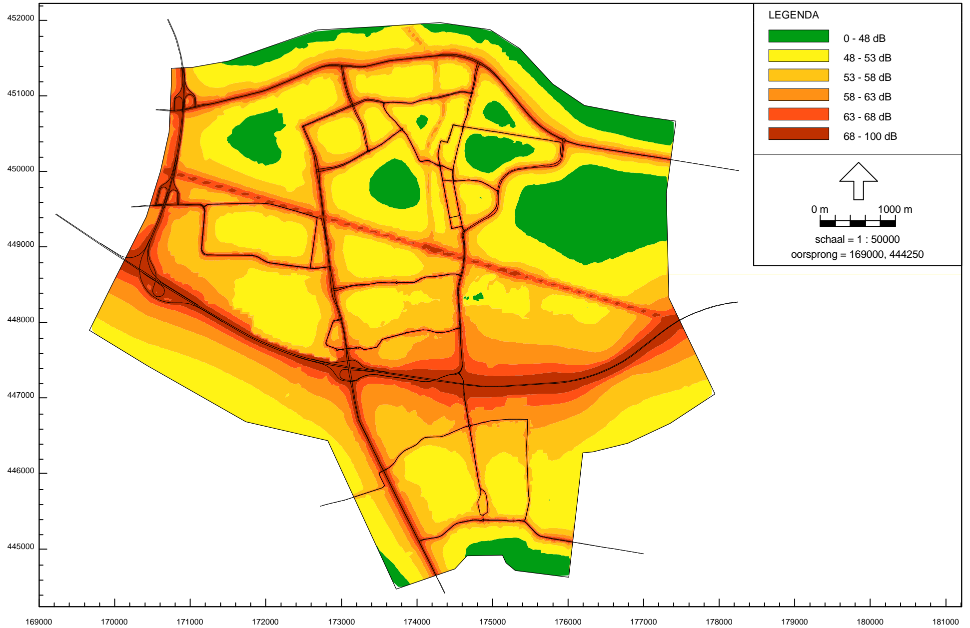
Situatie: Alternatief minimaal ruimtebeslag 2020, gecumuleerd weg- en railverkeer (op basis Wgh2006) Geluidsbelastingen in Lden berekend op 5m hoogte
