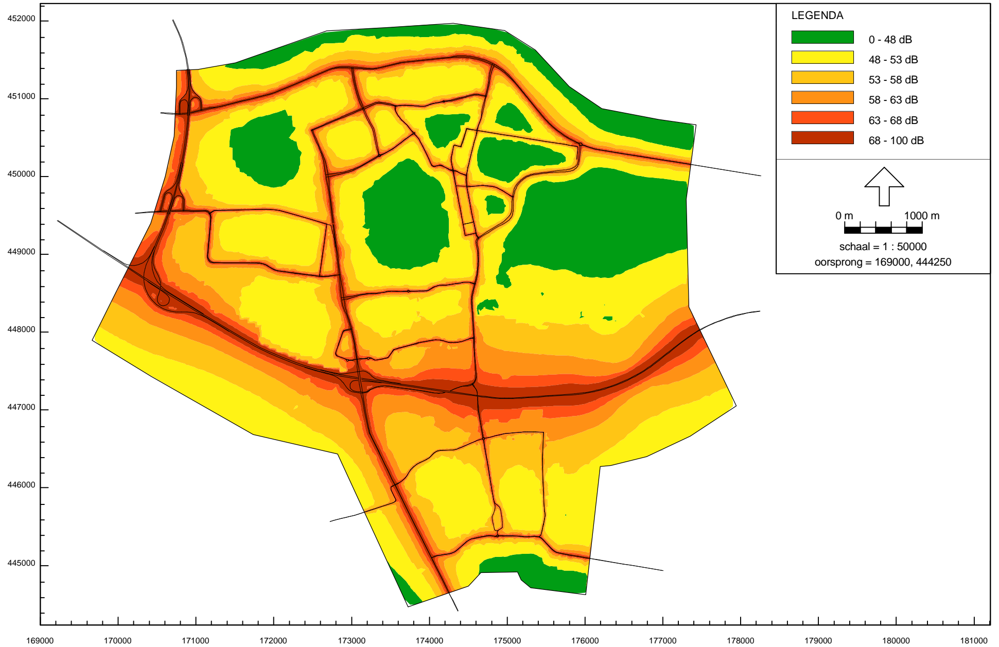
Situatie: Alternatief minimaal ruimtebeslag 2020, met maatregelen Parklaan Geluidsbelastingen in Lden berekend op 5m hoogte
