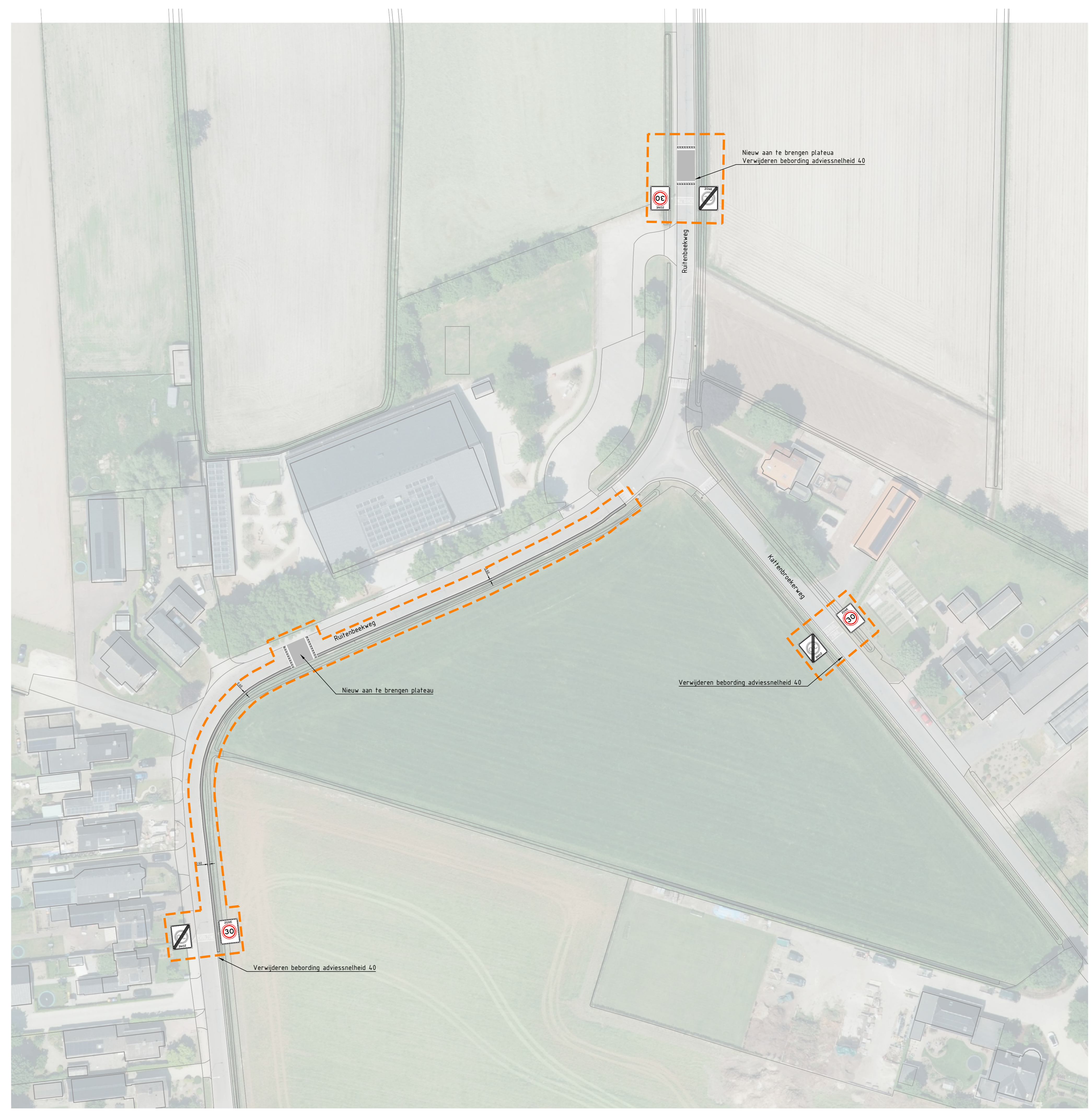
Ruitenbeekweg, Lunteren maatregel t.b.v. veiligheid fietsverkeer Schaal: 1:500
