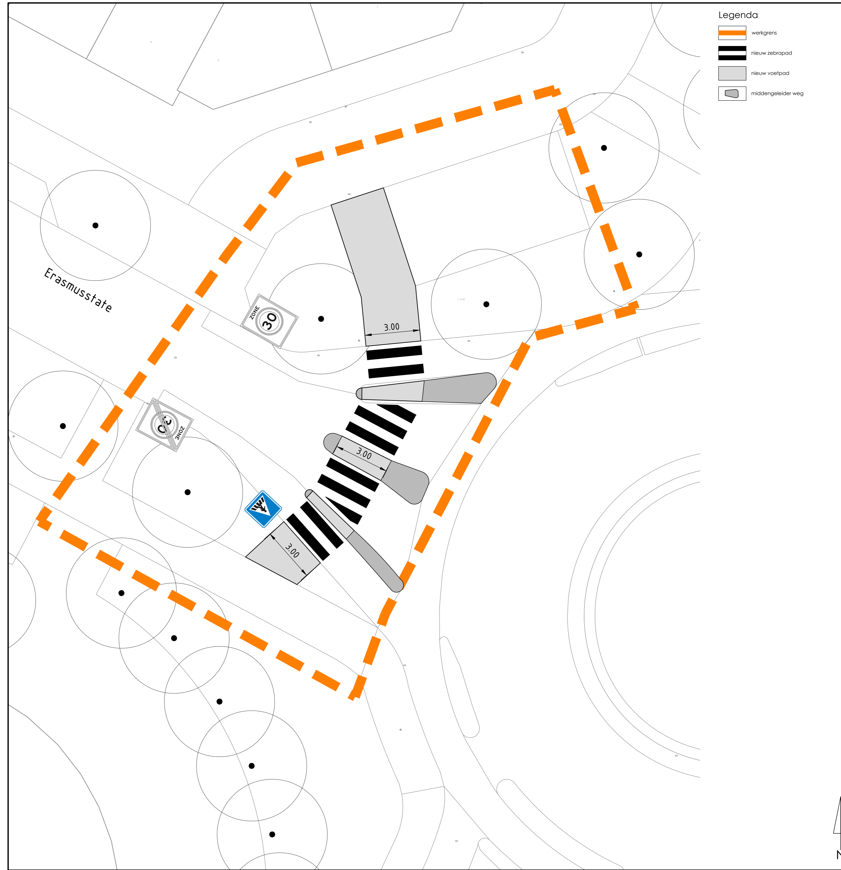
Erasmusstate - Laan der Verenigde Naties maatregel t.b.v. ondersteunende voetgangers Schaal: 1:100
