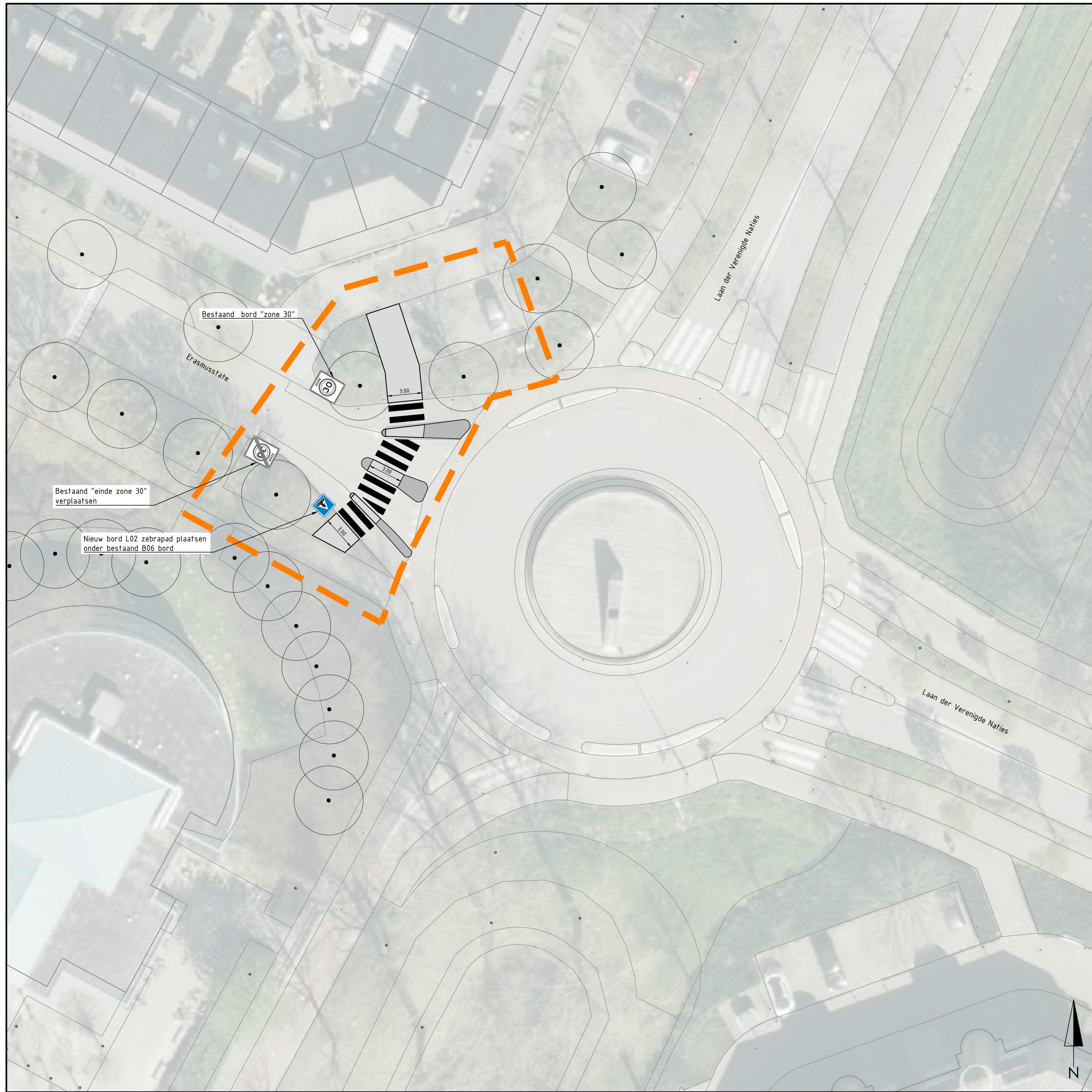
Erasmusstate - Laan der Verenigde Naties maatregel t.b.v. ondersteunende voetgangers Schaal: 1:200
