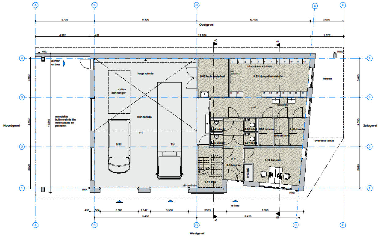
Begane grond
